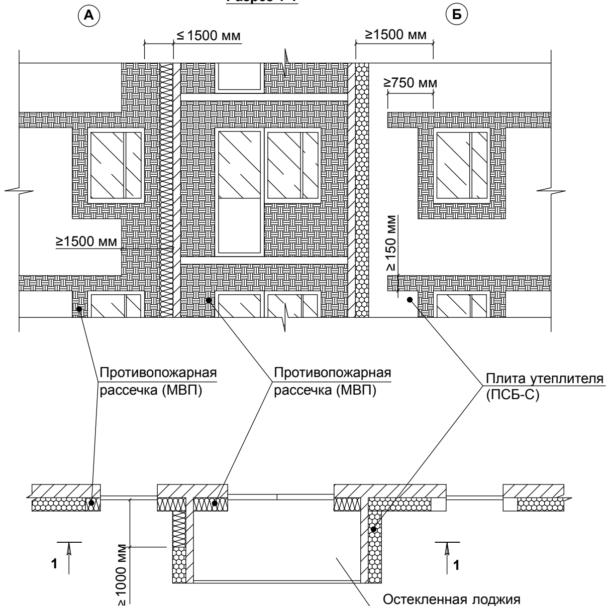
Разрез 1-1
